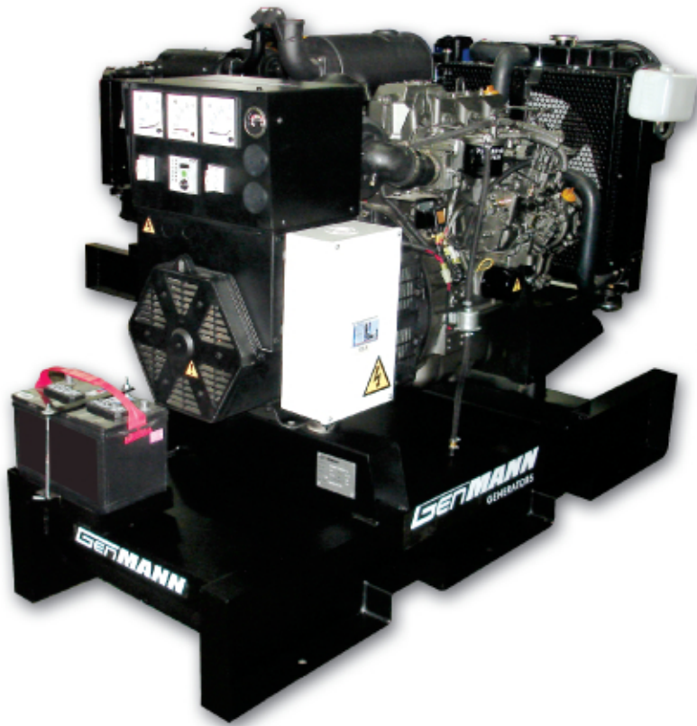
Planta Eléctrica Diesel 30KW Trifásico Diesel Generator Set 30KW Three Phase
